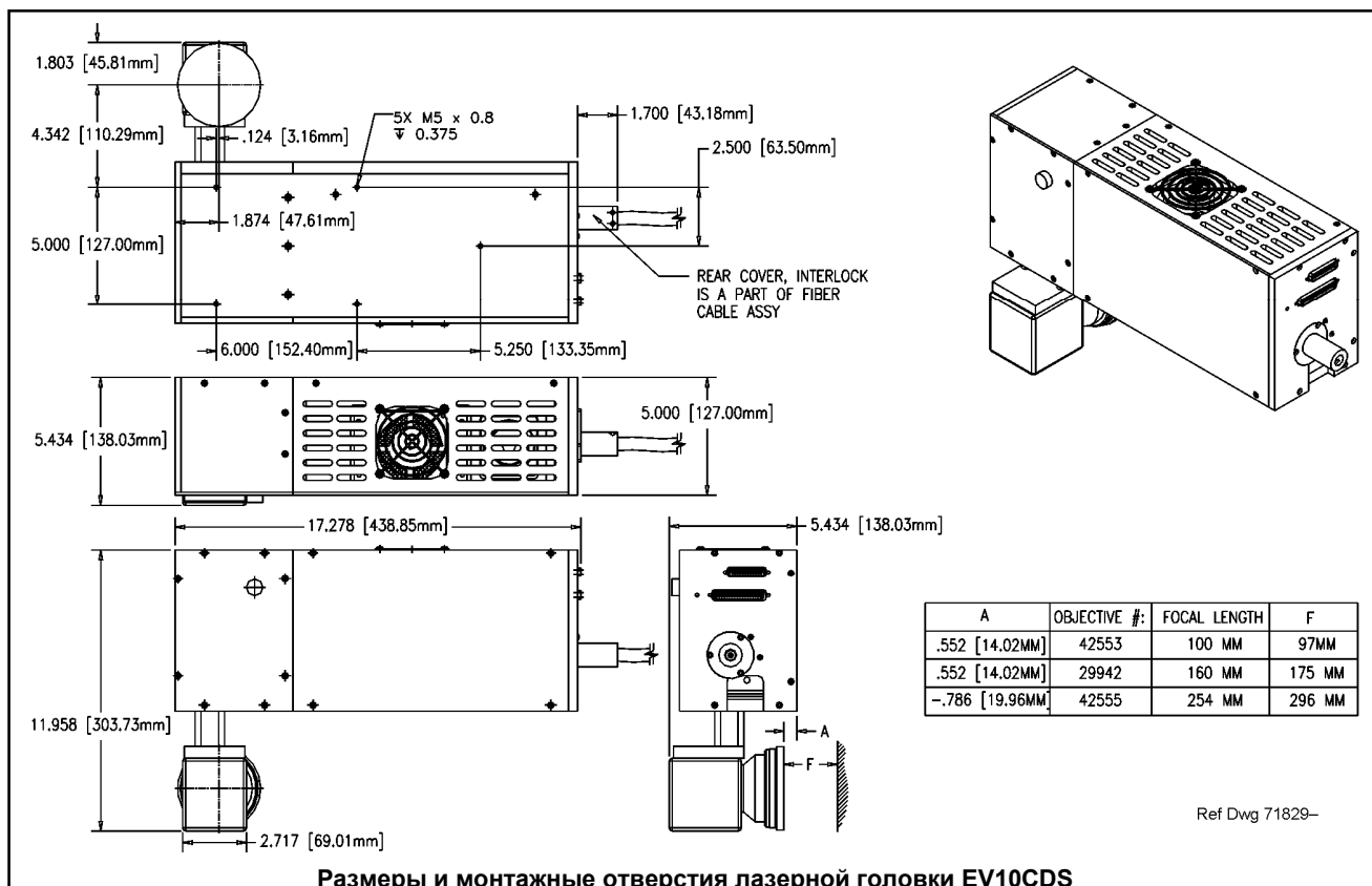
Размеры и монтажные отверстия лазерной головки EV10CDS
