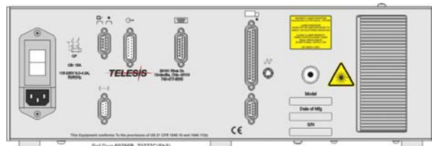
Контроллер E1015 Задняя панель – с внешним ПК
