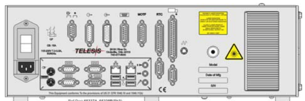
Контроллер E1015 Задняя панель – с встроенным ПК
